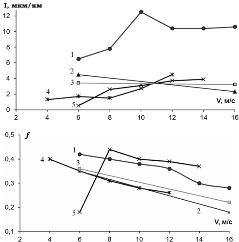
Рис. 4. Интенсивность изнашивания ( I ) и коэффициент трения ( f ) сплава ВК8 без покрытия (1) и с ЭИЛ-покрытиями в зависимости от скорости скольжения ( V ): TiNAIN c/c (2); TiNAIN б/с (3)Л; ТБНА20 (4), КНТ14А (5)
