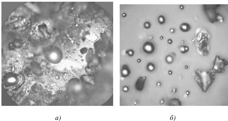
Рис. 1. Микроструктура рабочей поверхности анода (керамика на основе ZrB_2 ) после ЭИЛ сплава ВК6 (а) и продукты эрозии анода (б), \times 800 [14]
