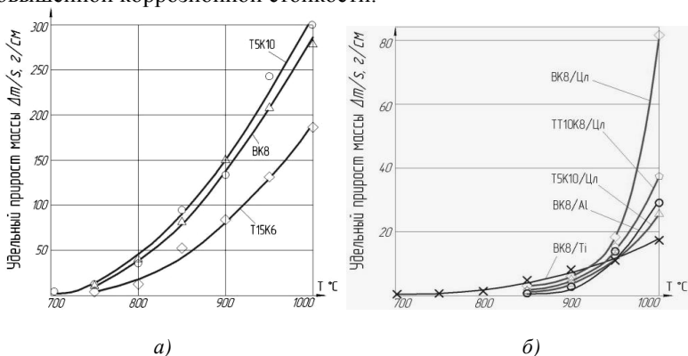
Рис. 2. Изменение с температурой удельного привеса образцов и ВТС при нагреве на воздухе со скоростью 20 °С/мин.:
