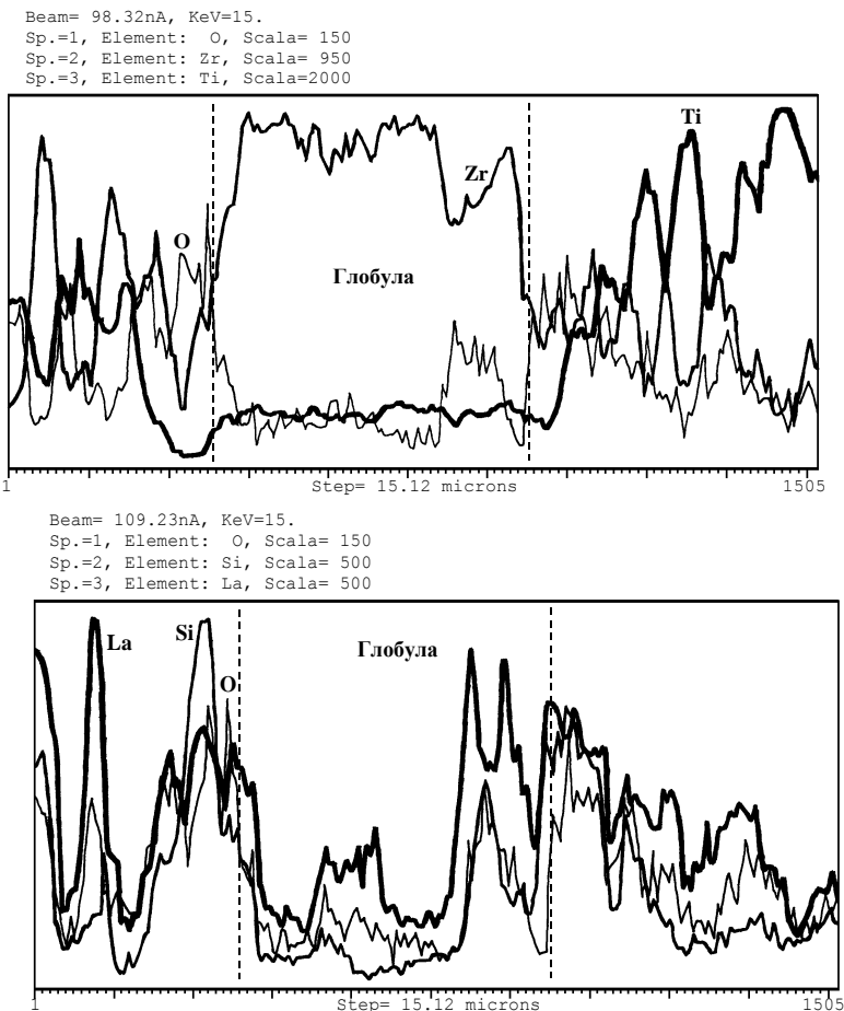
Рис. 3. Распределение элементов на поверхности ЭИЛ-покрытия с глобулярной структурой системы ЦЛАБ-2/ВТЗ-1 (основа) [12]
