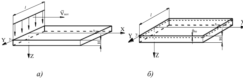
Рис. 1. Схема дії стрічкового електронного потоку на плоско-паралельну пластину (а) та розташування модифікованого ПШ (б)
